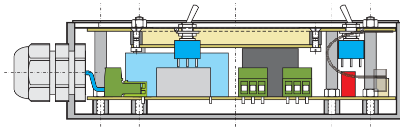
Querschnitt
