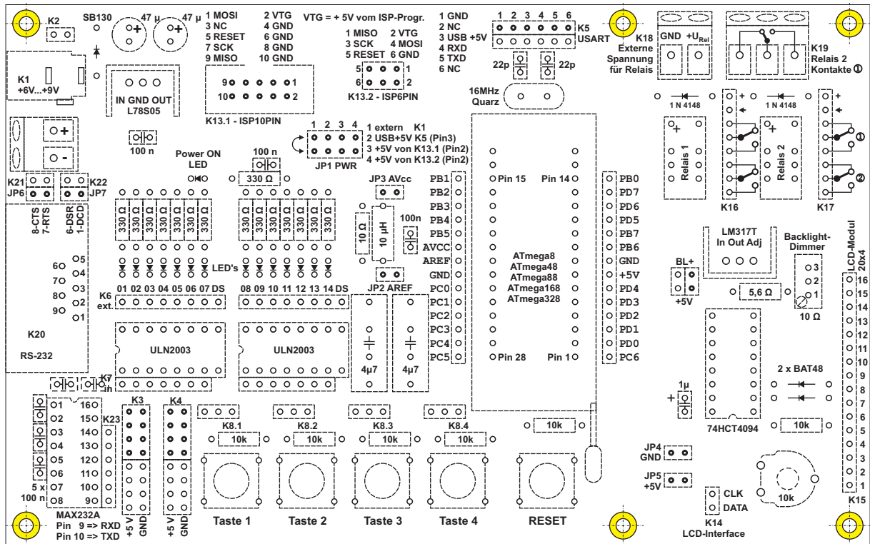
Beschaltungsseite; Maßstab 1:1
