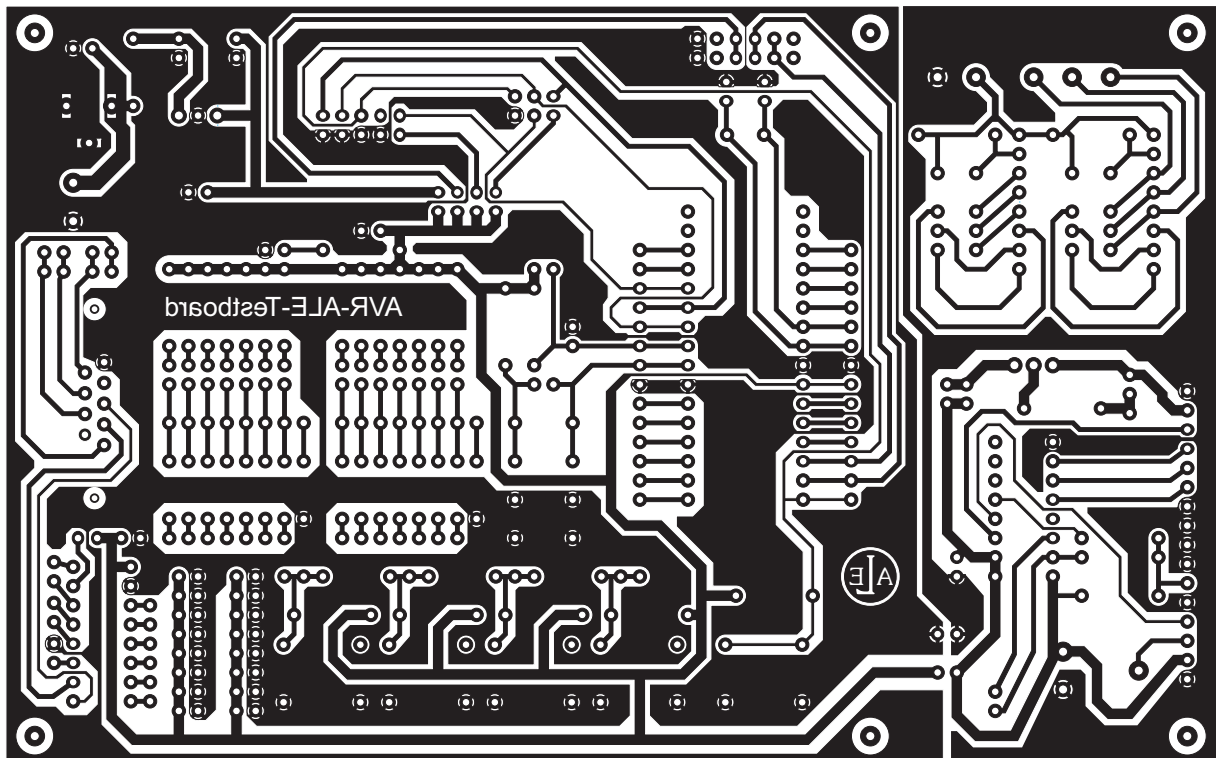
Lötseite (seitenverkehrt); Maßstab 1:1
